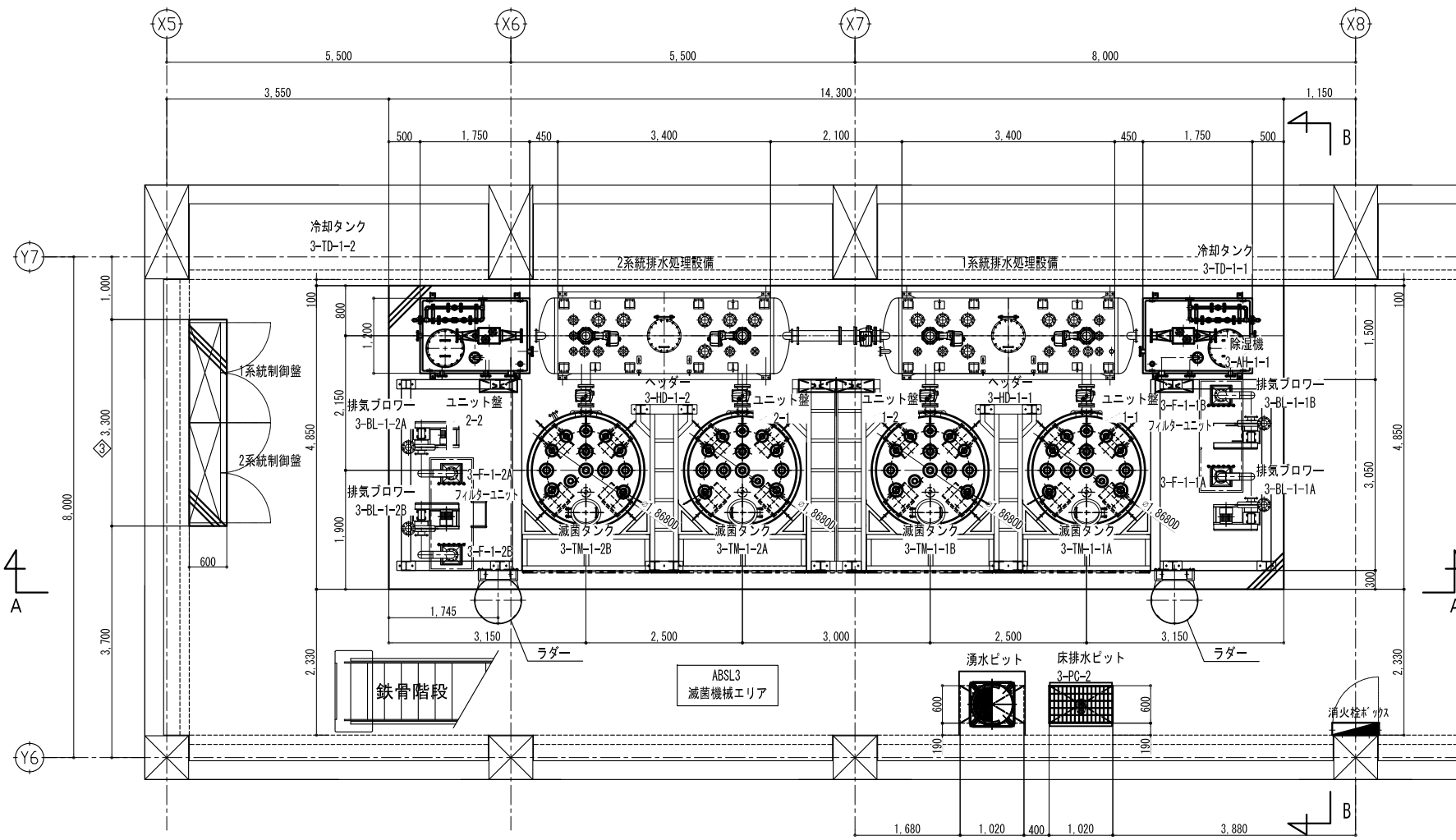
ABSL3機械室 平面図
