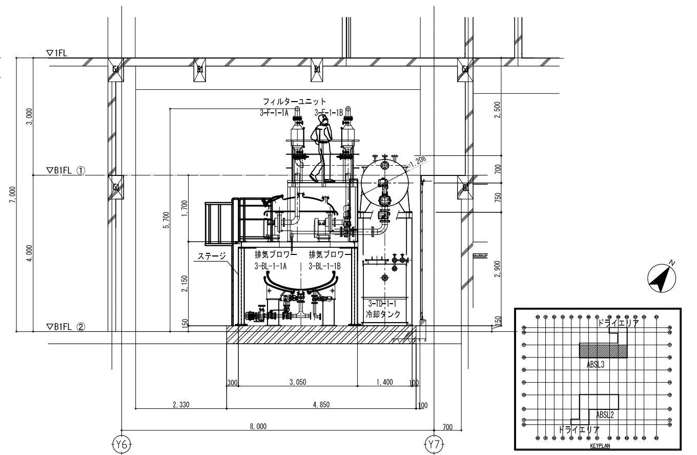
B-B断面図
