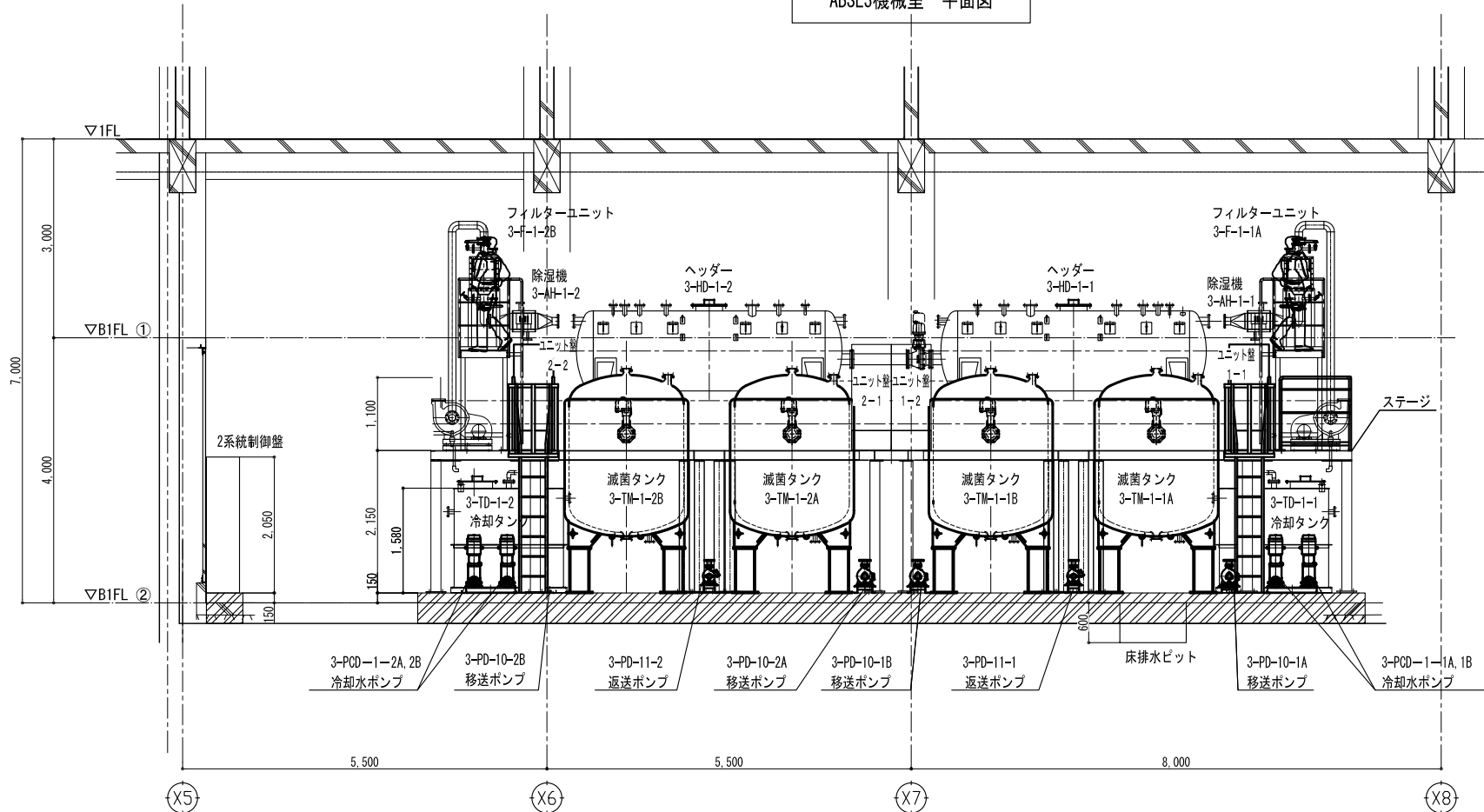
A-A断面図
